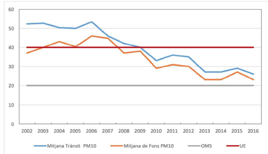
Figura 9. Evolució temporal de la mitjana anual agregada per estacions de trànsit i de fons de PM 10 (en µg/m 3 ) per al període 2002-2016
