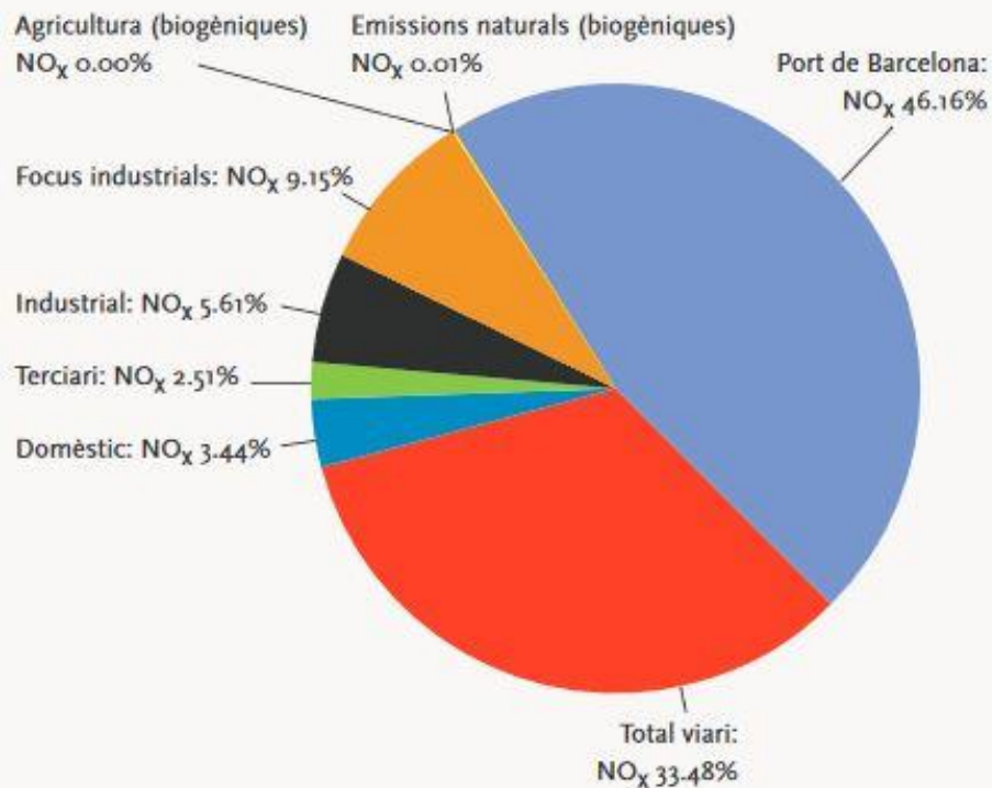
Distribució de les emissions d'NO x , a Barcelona, el 2013, per un total de 12.014 tones d'NO x
