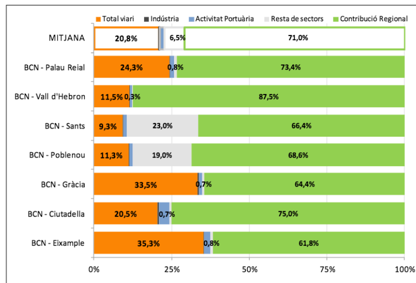
Gràfic 24: Origen de la contribució de la immissió de PM 10 segons el sector d'emissió - mitjana anual de l'any 2013.
