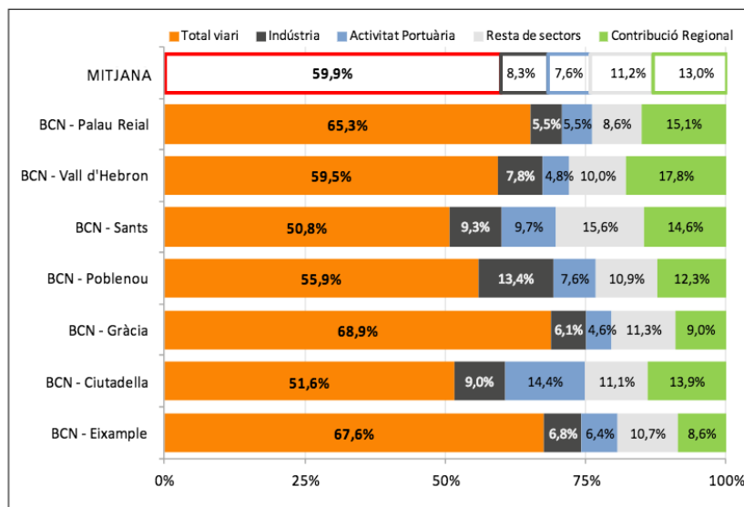
Gràfic 23: Origen de la contribució de la immissió d'NO 2 segons el sector d'emissió i la mitjana anual de l'any 2013.
